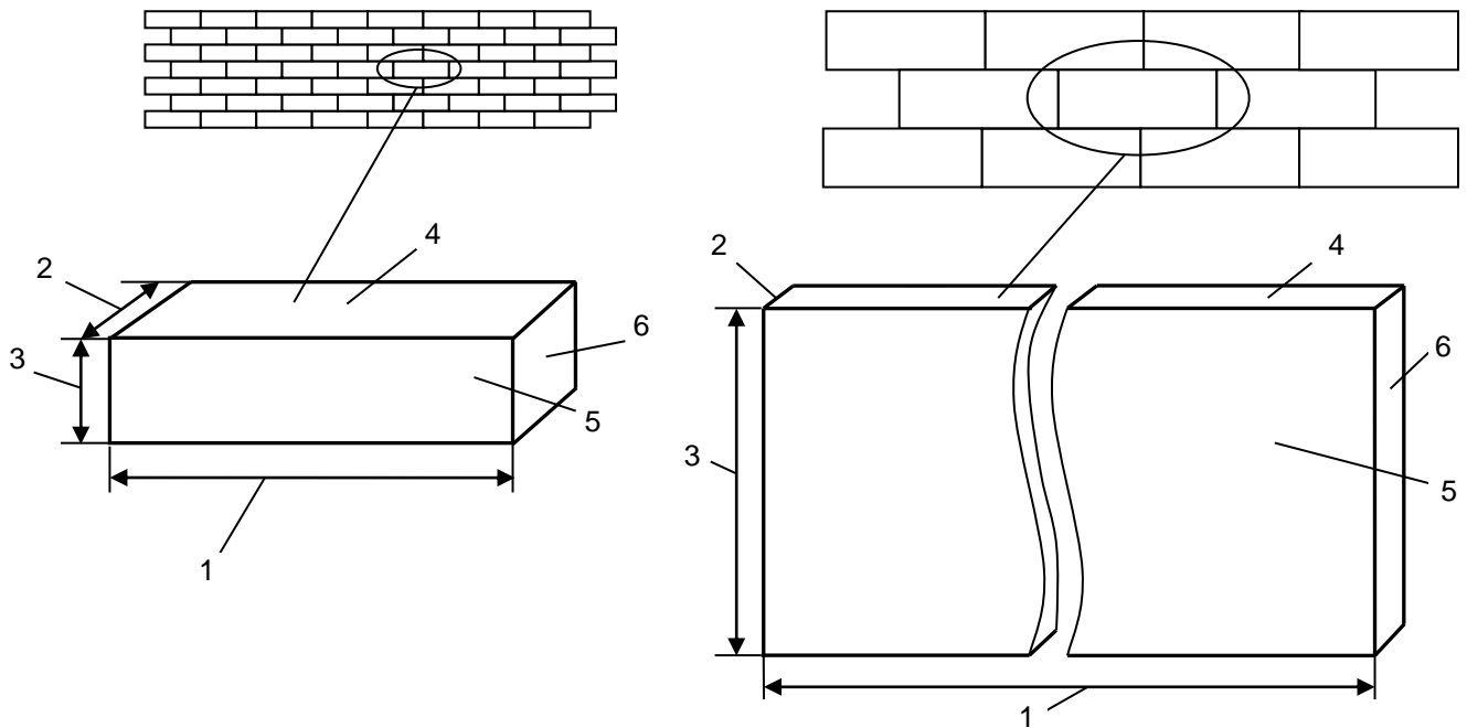
A. Bê tông khí chưng áp dạng khối (AACB)
